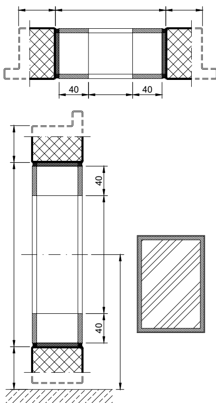
Flächenbündige Verglasung
