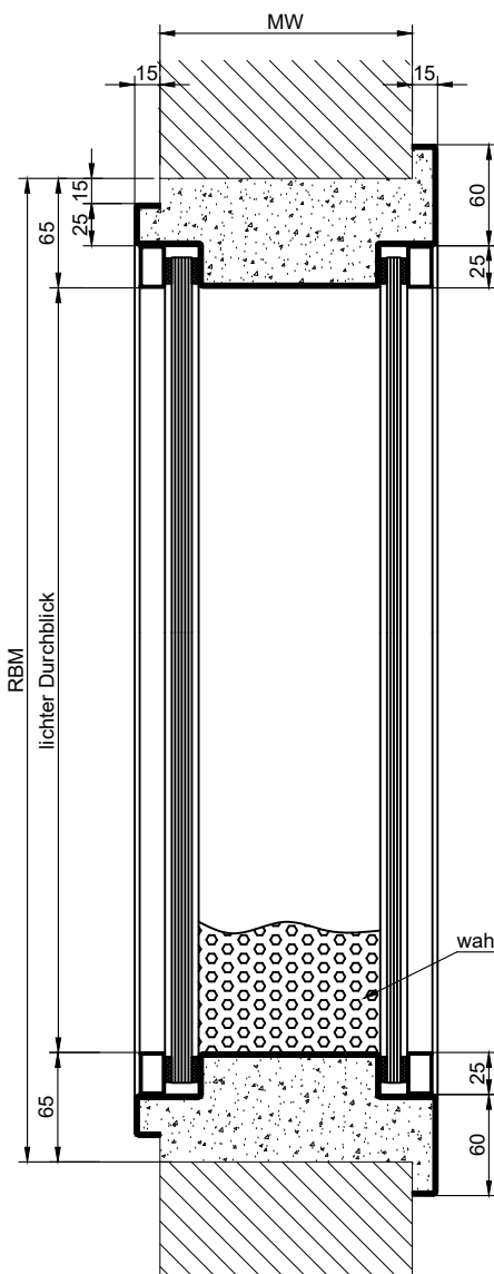
Umfassungszarge
