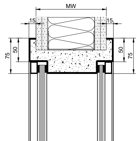
2-teilige Umfassungszarge
