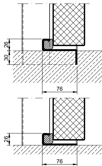
Anschlagschwelle mit Absenkdrichtung
