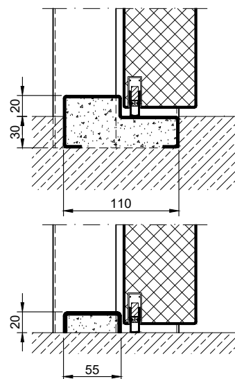
Vollschwelle
