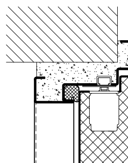
Integrierter Türschließer
