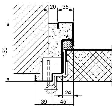
Objektbänder VB-3D
