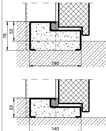
Vollschwelle
